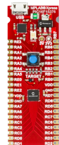
MPLAB® Xpress PIC16F15376 评估板 (部件编号: DM164143)
