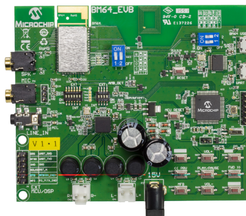
BM64 Bluetooth音频评估板 (BM-64-EVB-C2)
