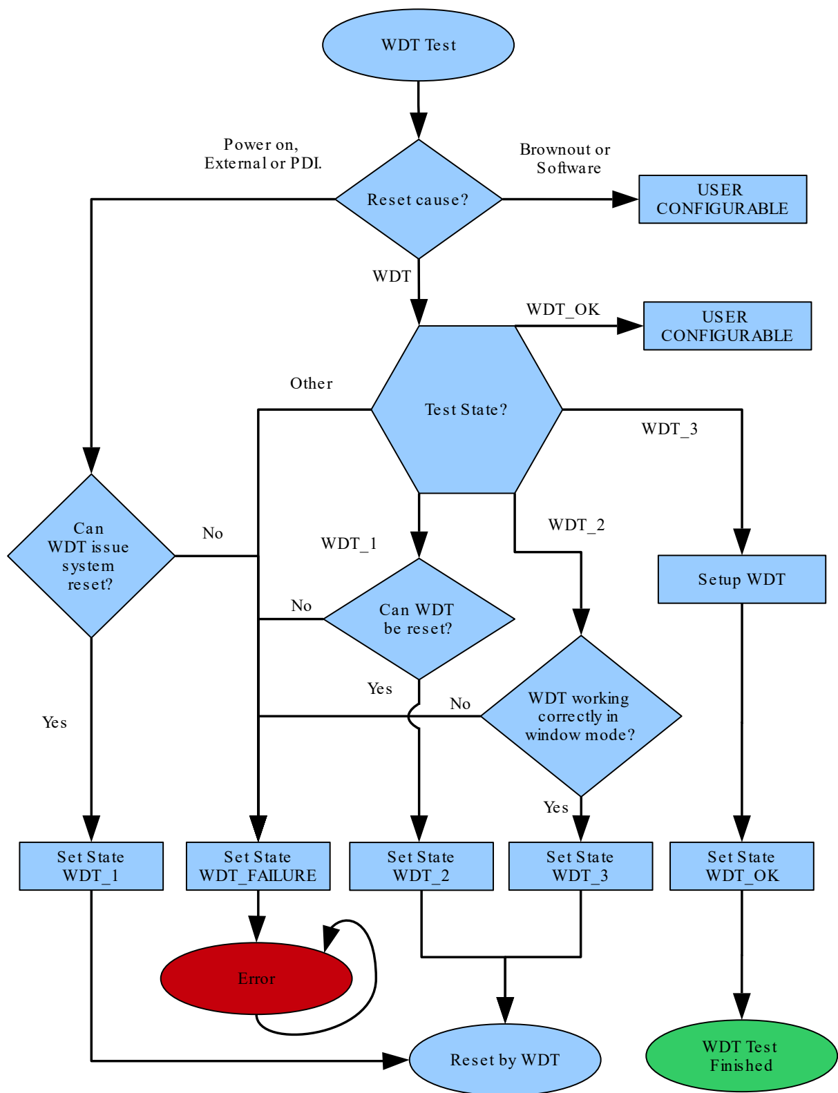
图 6-1. 看门狗测试
